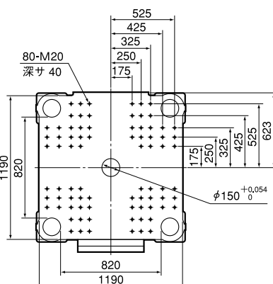
固定盤
