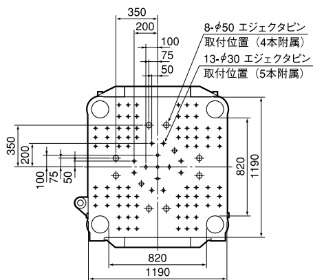
可動盤
